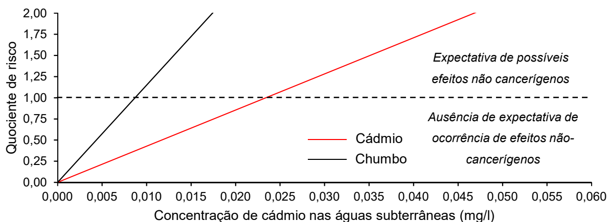
Figura 6.19 - Variação do quociente de risco não cancerígeno com a concentração de chumbo e cádmio
