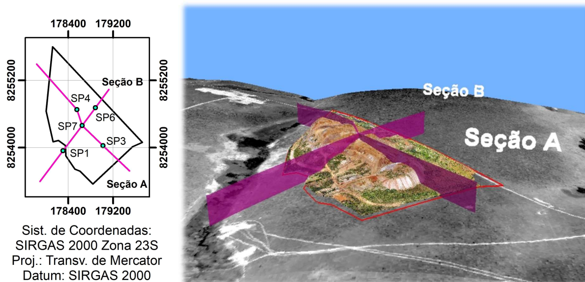
Figura 6.3 – Croqui de localização das seções realizadas e das sondagens de Pereira et al. (1997) e representação dessas seções no modelo tridimensional.
