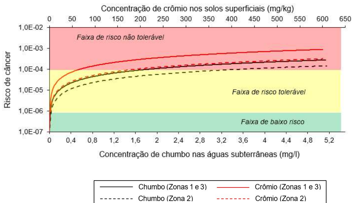
Figura 6.20 – Variação do risco de câncer com a concentração de chumbo e cromo.
