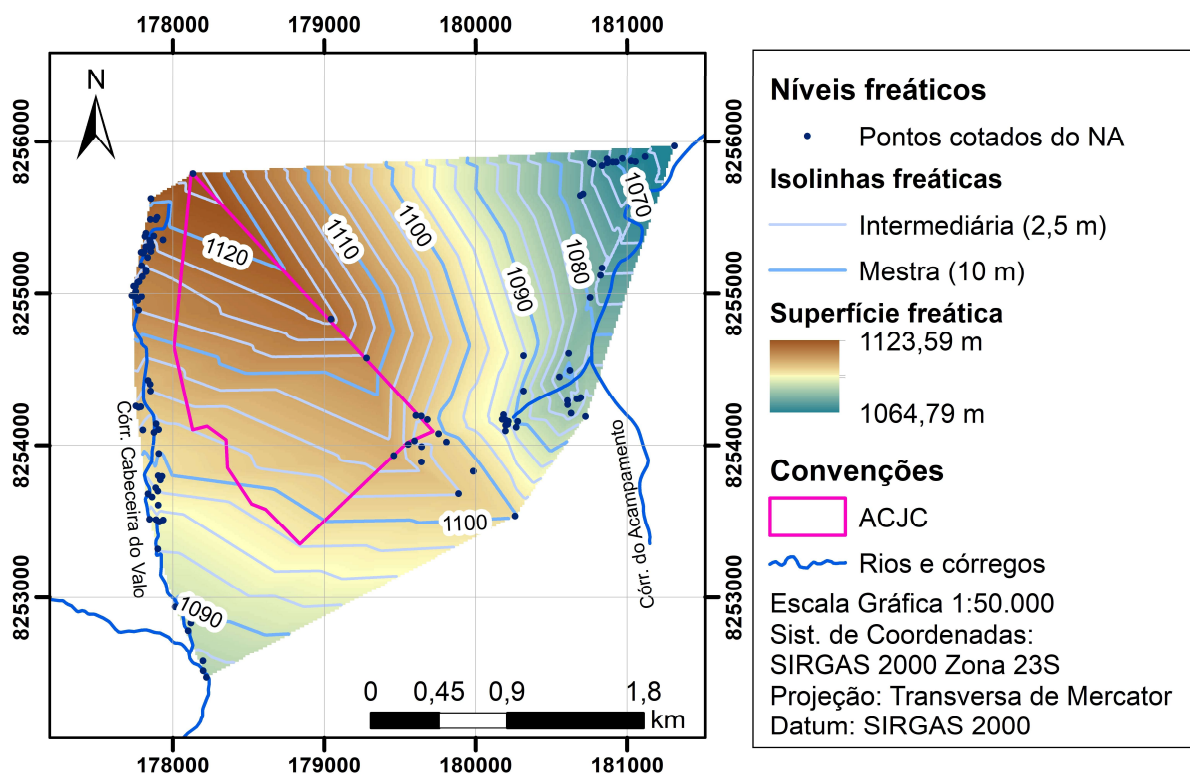
Figura 6.2 – Superfície freática e isolinhas correlatas obtidas por Stollberg & Weiß (2011).
