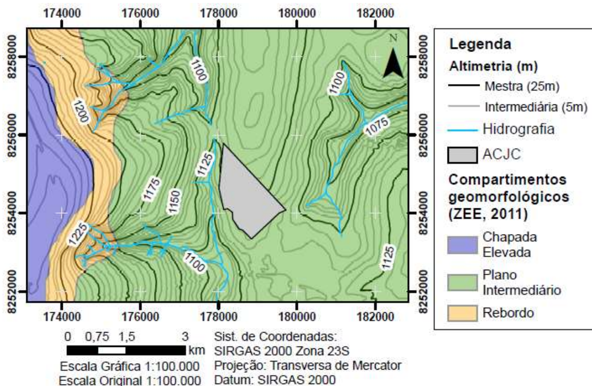
Figura 4.10 – Altimetria e compartimentação geomorfológica nas adjacências do ACJC.
