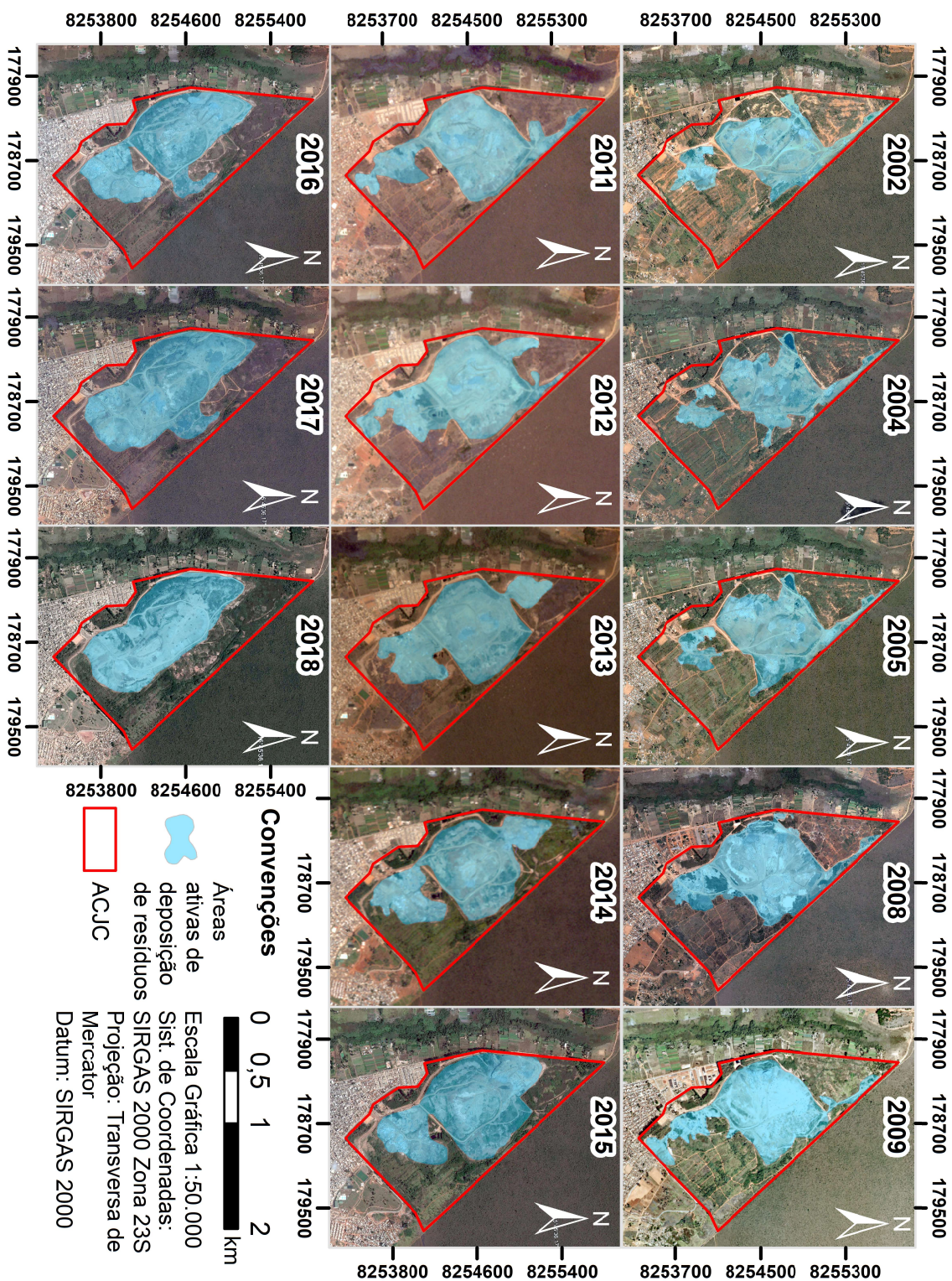
Figura 4.3 – Evolução da disposição de resíduos no ACJC entre 2002 e 2018.
