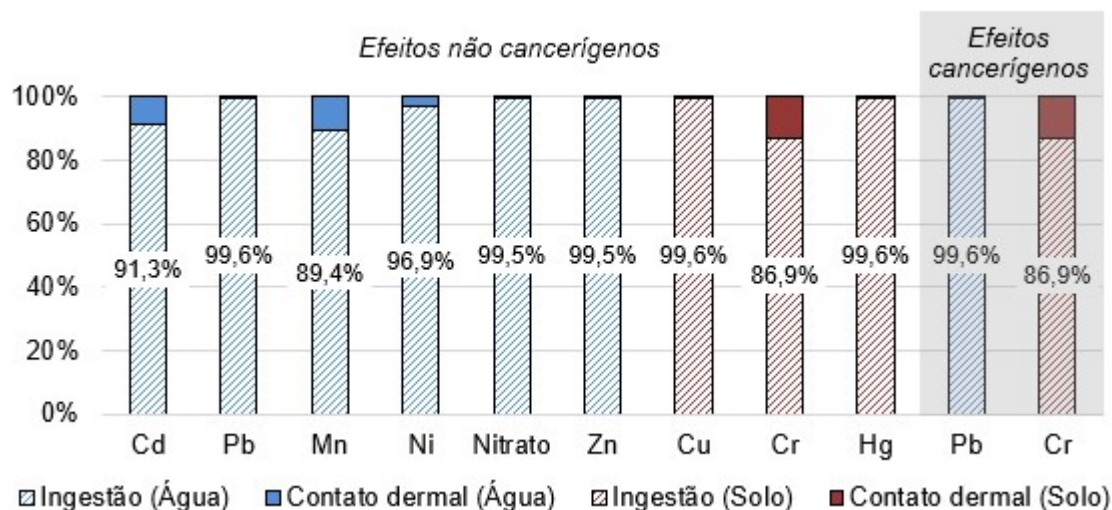
Figura 6.17 – Contribuição percentual média dos caminhos de exposição para os valores de QR_{total} e SF_{total} .
