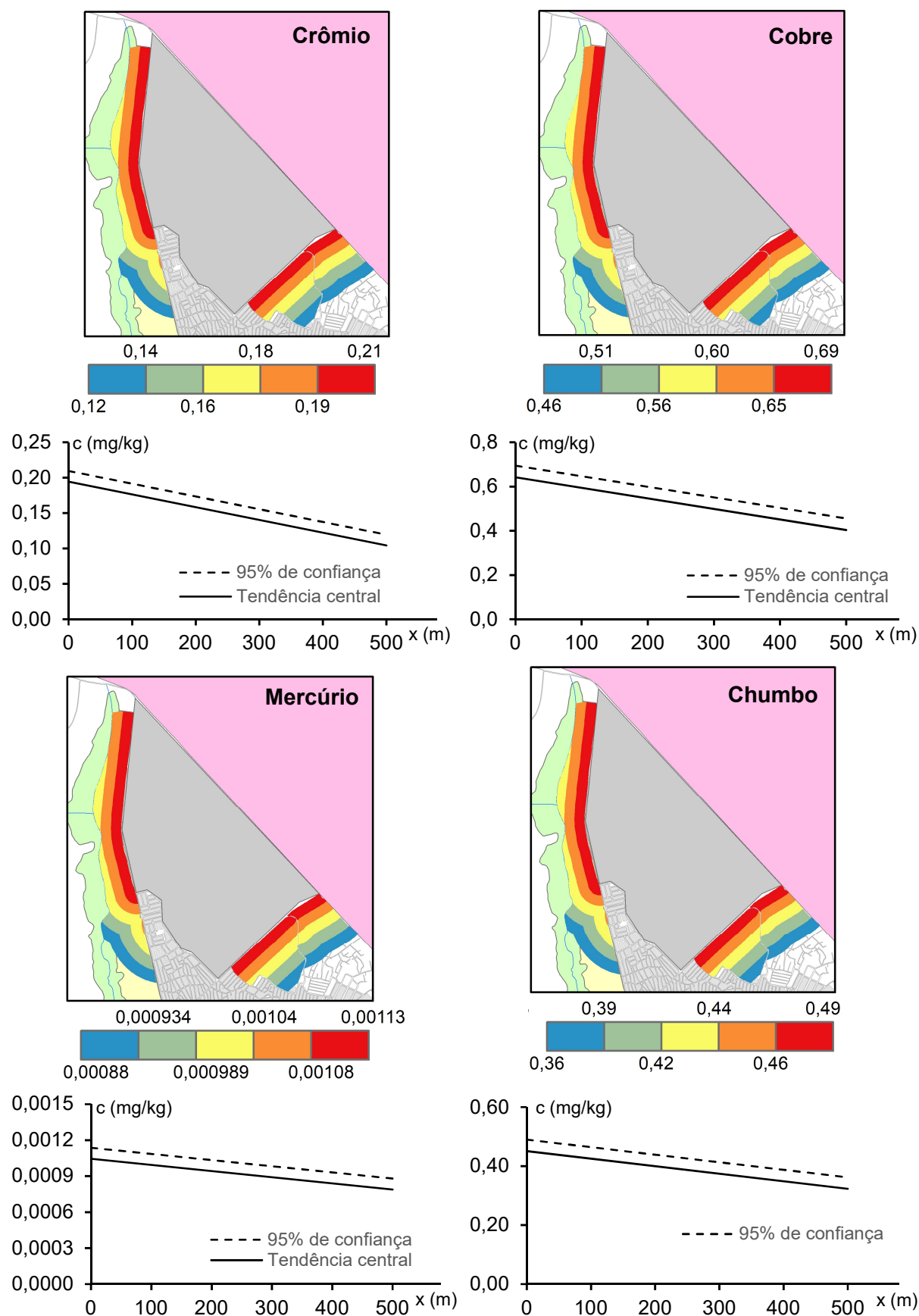
Figura 6.16 – Cenários de contaminação referentes a zona não saturada (solos superficiais)
