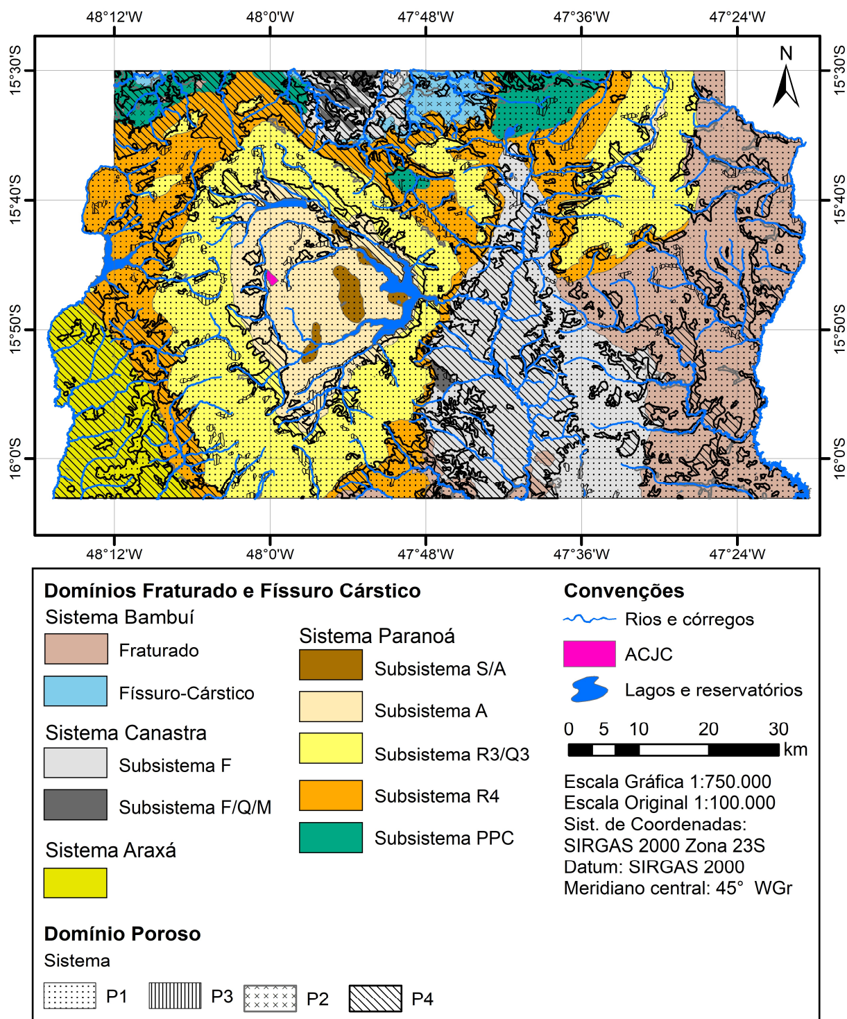
Figura 4.16 – Mapa hidrogeológico do Distrito Federal. Fonte: ZEE (2011)
