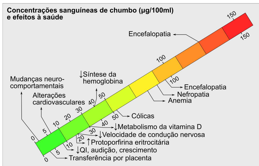
Figura 6.18 – Efeitos à saúde humana relacionados à concentração sanguínea de chumbo. Adaptado de OEHHA (2009)
