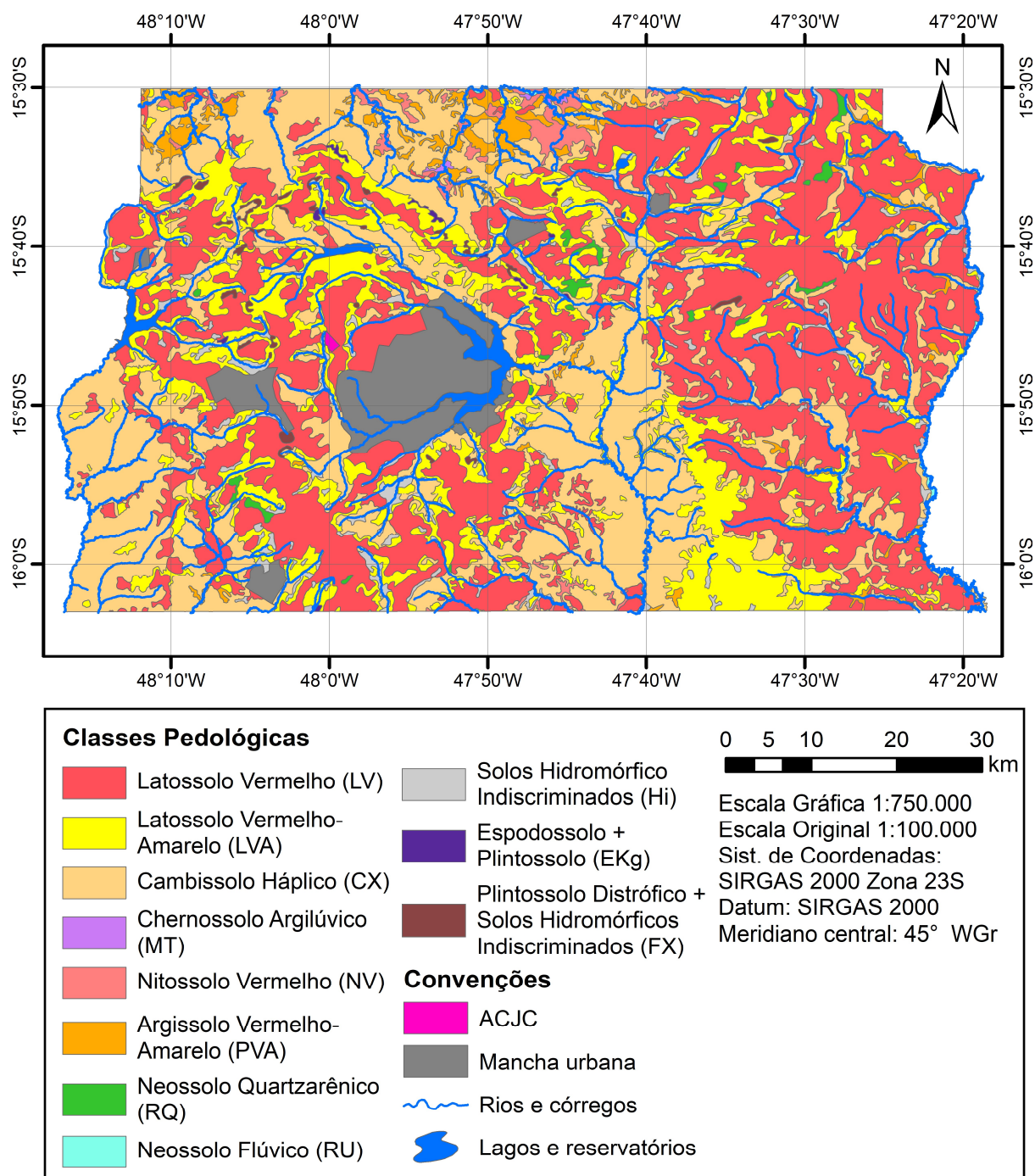
Figura 4.14 – Mapa pedológico do Distrito Federal. Dado de Reatto et al. (2004)
